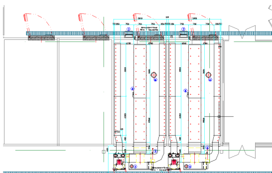
Grundrissplan
